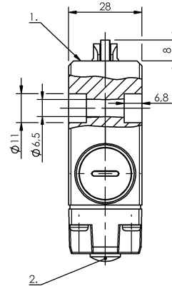
1) Опорная кромка 2) Функциональный индикатор FD/FE/LL
