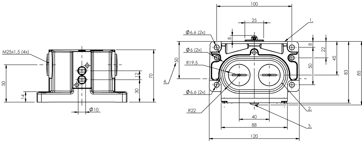
1) Опорная кромка 2) Функциональный индикатор FD/FE/LL 3) Уплотнительное кольцо 4) Кабельный ввод
