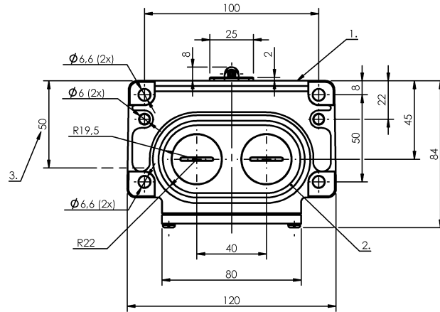
1) Опорная кромка 2) Уплотнительное кольцо 3) Кабельный ввод
