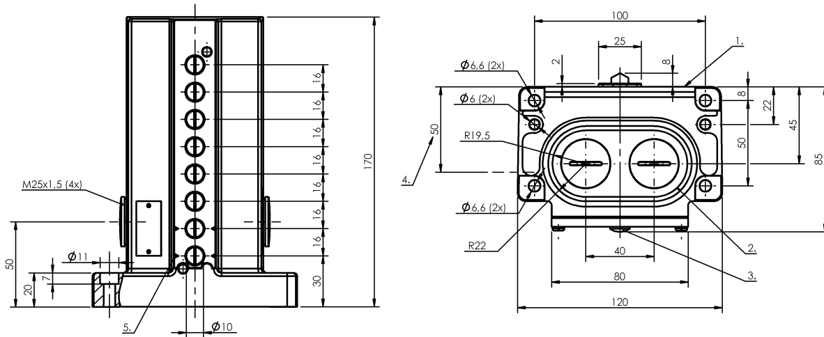
1) Опорная кромка 2) Уплотнительное кольцо 3) Функциональный индикатор FD/FE/LL 4) Кабельный ввод 5) Марк. Предопр. точка коммутации
