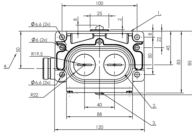
1) Опорная кромка 2) Уплотнительное кольцо 3) Функциональный индикатор FD/FE/LL 4) Кабельный ввод
