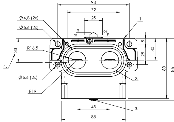
1) Опорная кромка 2) Уплотнительное кольцо 3) Функциональный индикатор FD/FE/LL 4) Кабельный ввод 5) Марк. Предохран. точка коммутации
