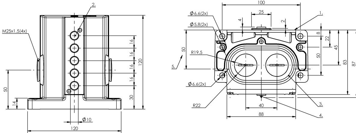
1) Опорная кромка 2) Активная поверхность 3) Уплотнительное кольцо 4) Функциональный индикатор FD/FE/LL 5) Кабельный ввод
