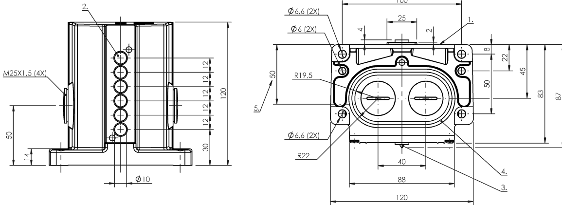
1) Опорная кромка 2) Активная поверхность 3) Функциональный индикатор FD/FE/LL 4) Уплотнительное кольцо 5) Кабельный ввод
