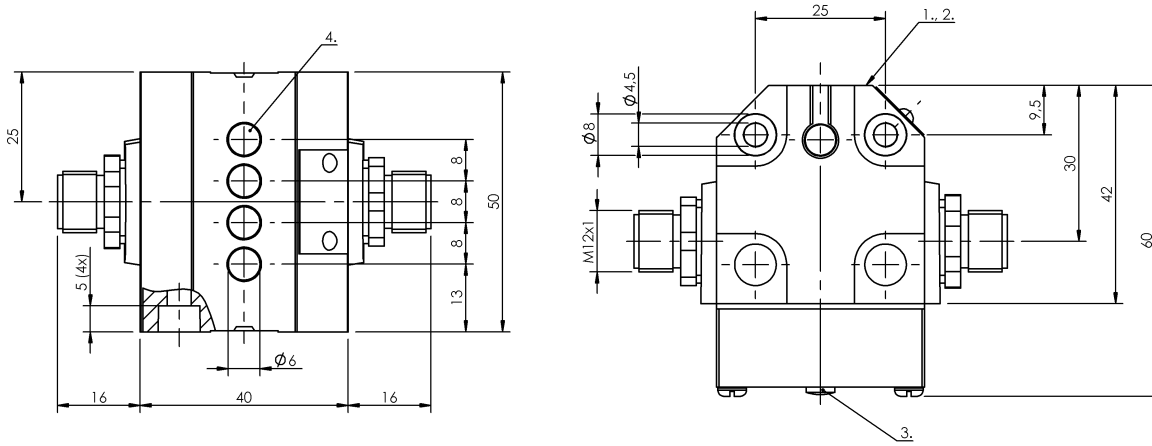
1) Опорная кромка 2) Активная поверхность 3) Функциональный индикатор FD/FE/LL 4) 1-я точка коммутации
