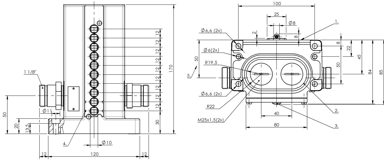
1) Опорная кромка 2) Уплотнительное кольцо 3) Функциональный индикатор FD/FE/LL 4) Марк. Предохран. точка коммутации 5) Кабельный ввод
