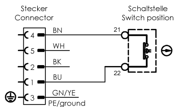
PE mit Gehäuse verbunden ground connected to housing
