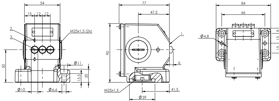
1) Опорная кромка 2) Марк. Предопр. точка коммутации 3) 1-я точка коммутации
