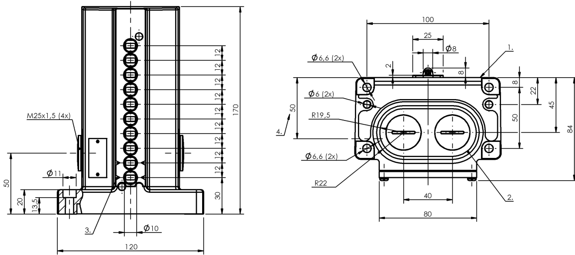
1) Опорная кромка 2) Уплотнительное кольцо 3) Марк. Предохран. точка коммутации 4) Кабельный ввод
