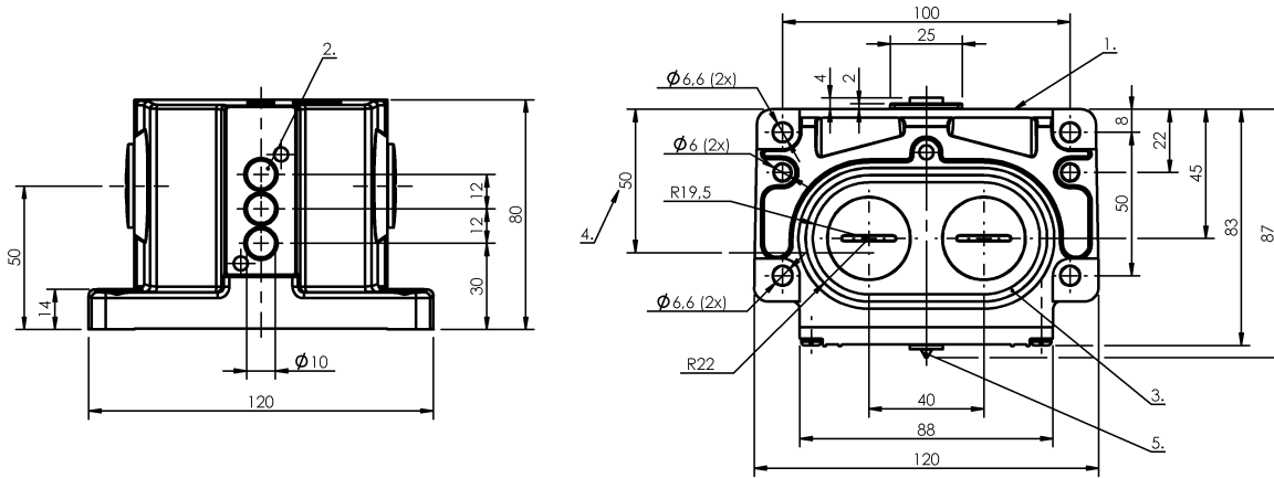
1) Опорная кромка 2) Активная поверхность 3) Уплотнительное кольцо 4) Кабельный ввод 5) Функциональный индикатор FD/FE/LL
