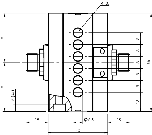
1) Опорная кромка 2) Функциональный индикатор FD/FE/LL 3) 1-я точка коммутации 4) Активная поверхность
