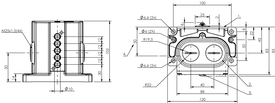
1) Опорная кромка 2) Уплотнительное кольцо 3) Функциональный индикатор FD/FE/LL 4) Кабельный ввод
