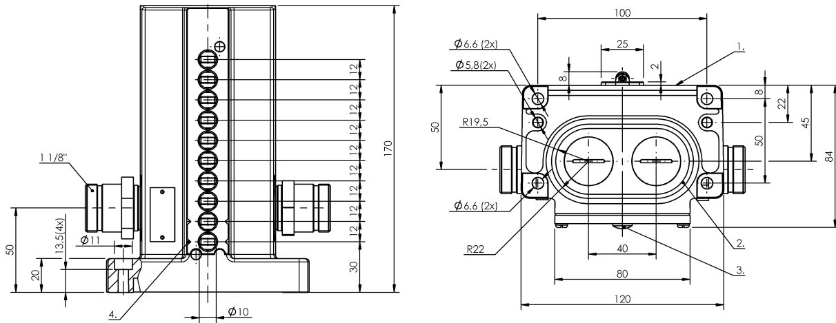
1) Опорная кромка 2) Уплотнительное кольцо 3) Функциональный индикатор FD/FE/LL 4) Марк. Предохран. точка коммутации
