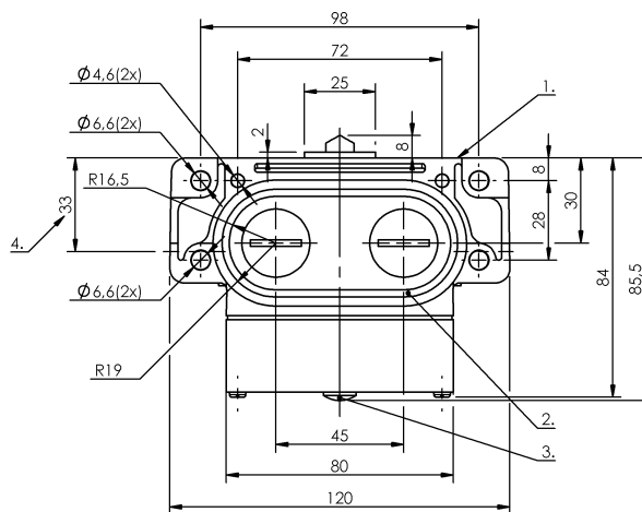
1) Опорная кромка 2) Уплотнительное кольцо 3) Функциональный индикатор FD/FE/LL 4) Кабельный ввод
