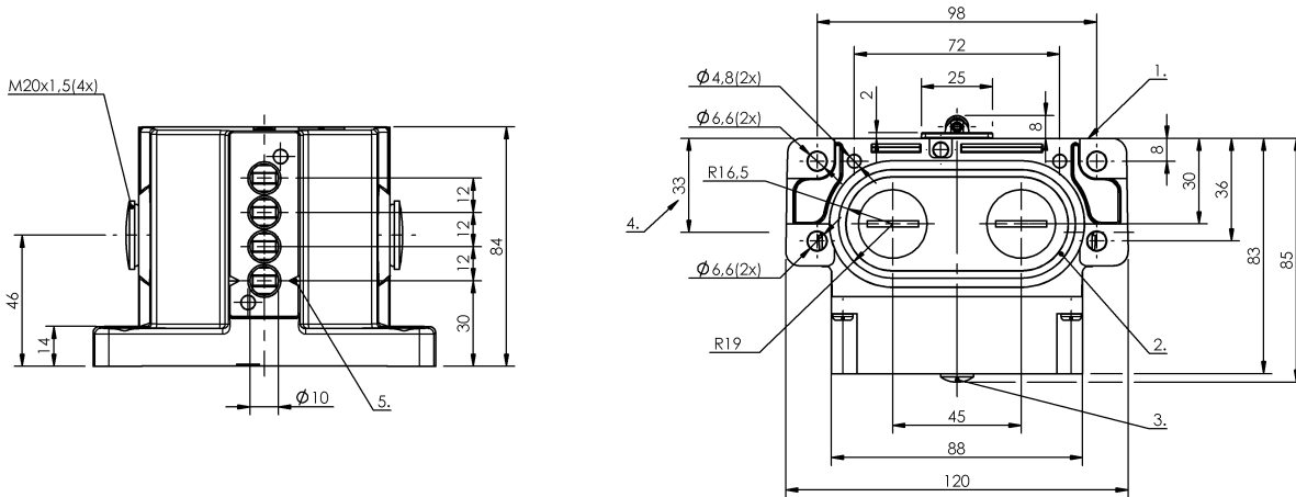
1) Опорная кромка 2) Уплотнительное кольцо 3) Функциональный индикатор FD/FE/LL 4) Кабельный ввод 5) Марк. Предохран. точка коммутации
