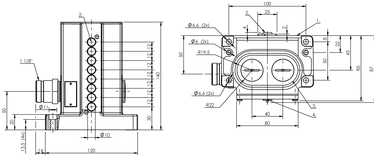
1) Опорная кромка 2) Активная поверхность 3) Уплотнительное кольцо 4) Функциональный индикатор FD/FE/LL
