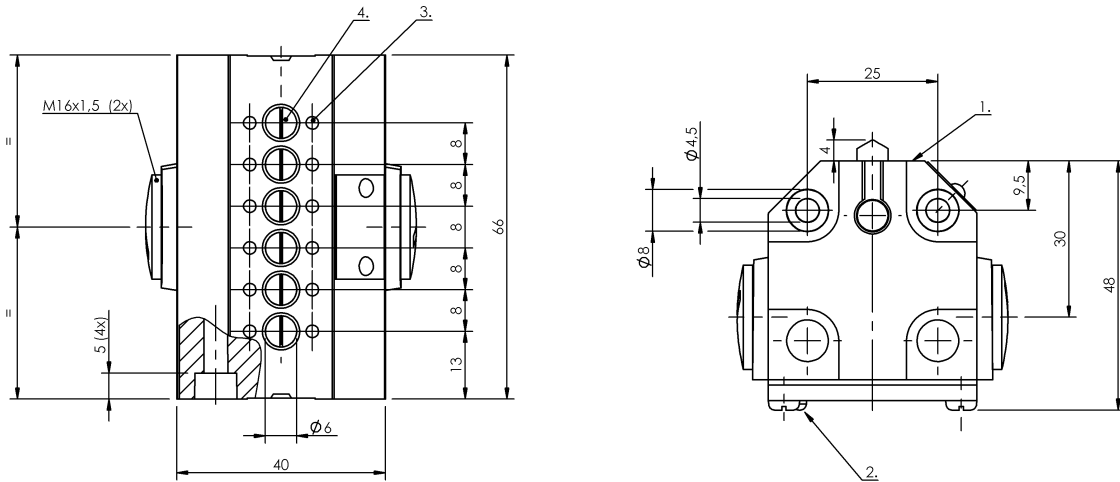
1) Опорная кромка 2) Функциональный индикатор FC 3) Марк. Предохран. точка коммутации 4) 1-я точка коммутации
