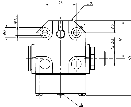
1) Опорная кромка 2) Активная поверхность 3) Функциональный индикатор FD/FE/LL 4) 1-я точка коммутации
