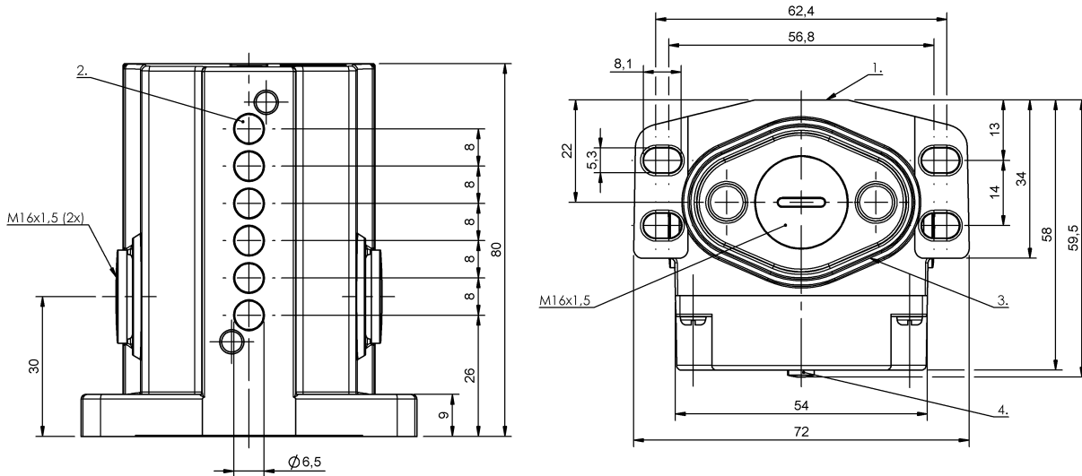
1) Опорная кромка 2) Активная поверхность 3) Уплотнительное кольцо 4) Функциональный индикатор FD/FE/LL
