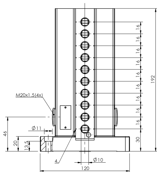
1) Опорная кромка 2) Уплотнительное кольцо 3) Кабельный ввод 4) Марк. Предохран. точка коммутации
