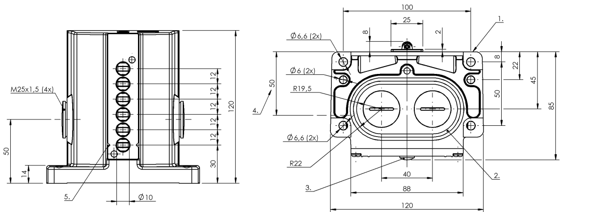
1) Опорная кромка 2) Уплотнительное кольцо 3) Функциональный индикатор FD/FE/LL 4) Кабельный ввод 5) Марк. Предохран. точка коммутации
