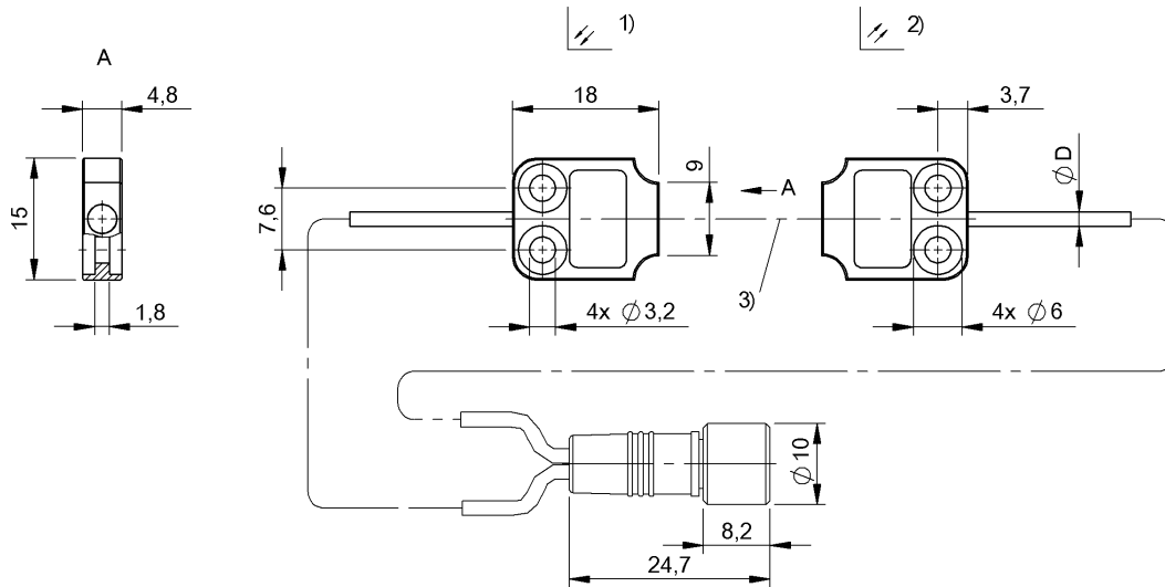
1) Передатчик 2) Приемник 3) Оптическая ось
