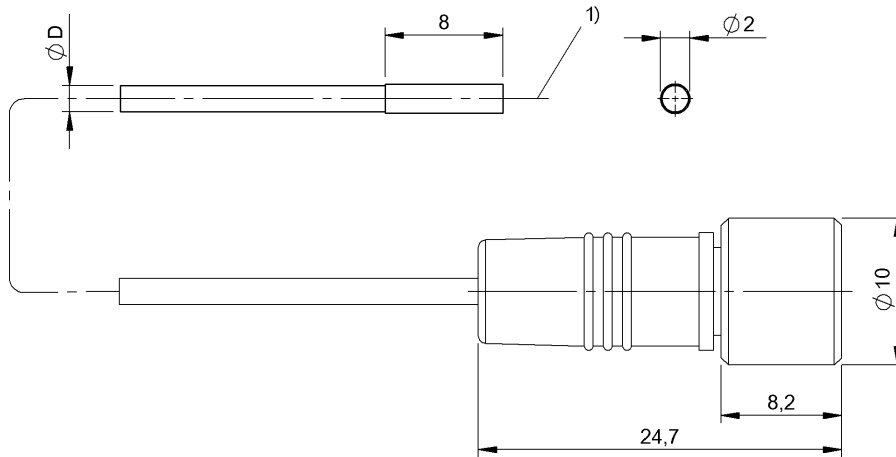
1) Оптическая ось
