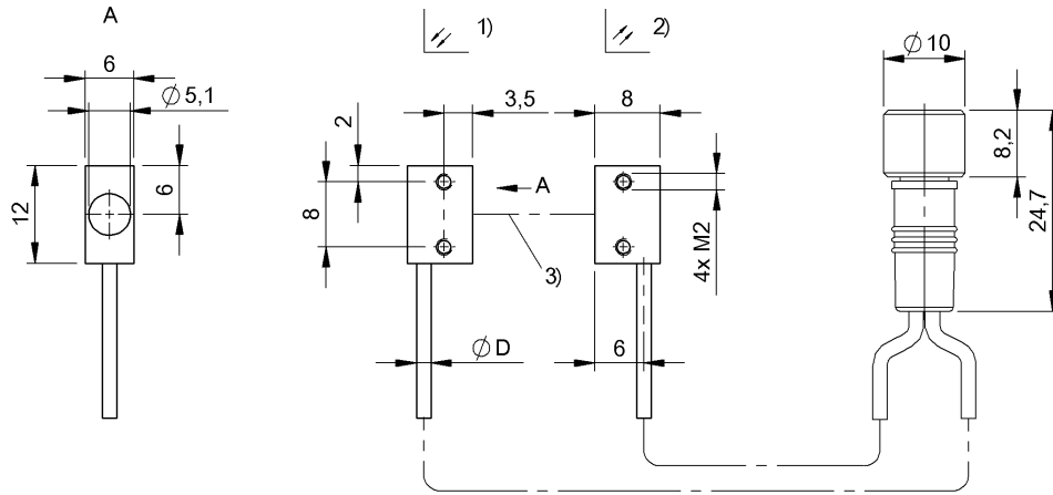
1) Передатчик 2) Приемник 3) Оптическая ось
