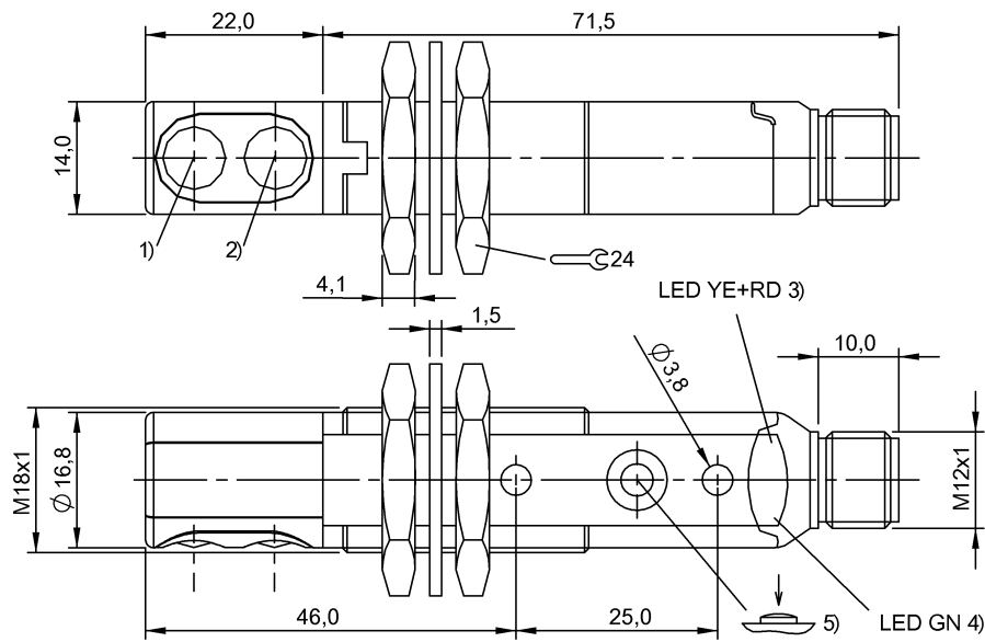
1) Оптическая ось, передатчик 2) Оптическая ось, приемник 3) Функция выхода 4) Стабильность / сбой 5) Sn
