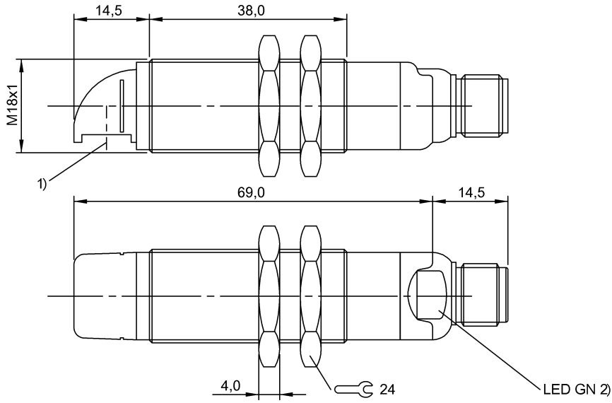
1) Оптическая ось 2) Напряжение питания
