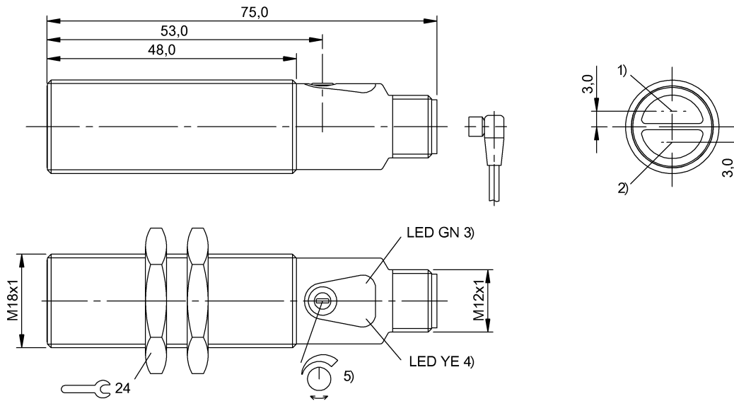
1) Оптическая ось, приемник 2) Оптическая ось, передатчик 3) Напряжение питания 4) Прием света / пограничная зона 5) Сигнал
