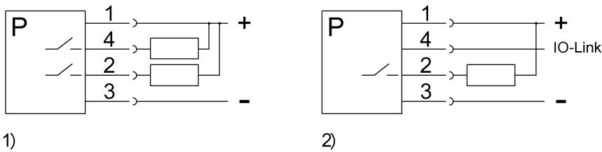
1) Стандартный режим 2) Режим IO-Link
