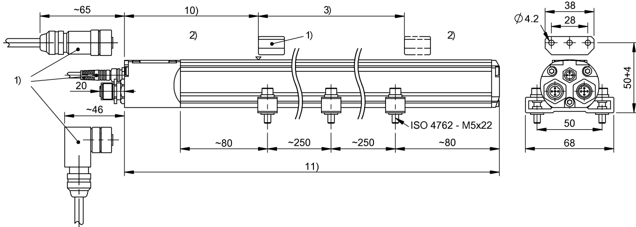
1) Не входит в комплект поставки 2) неиспользуемая область 3) Номинальная длина = измеряемая длина 10) Нулевая точка 11) Монтажная длина
