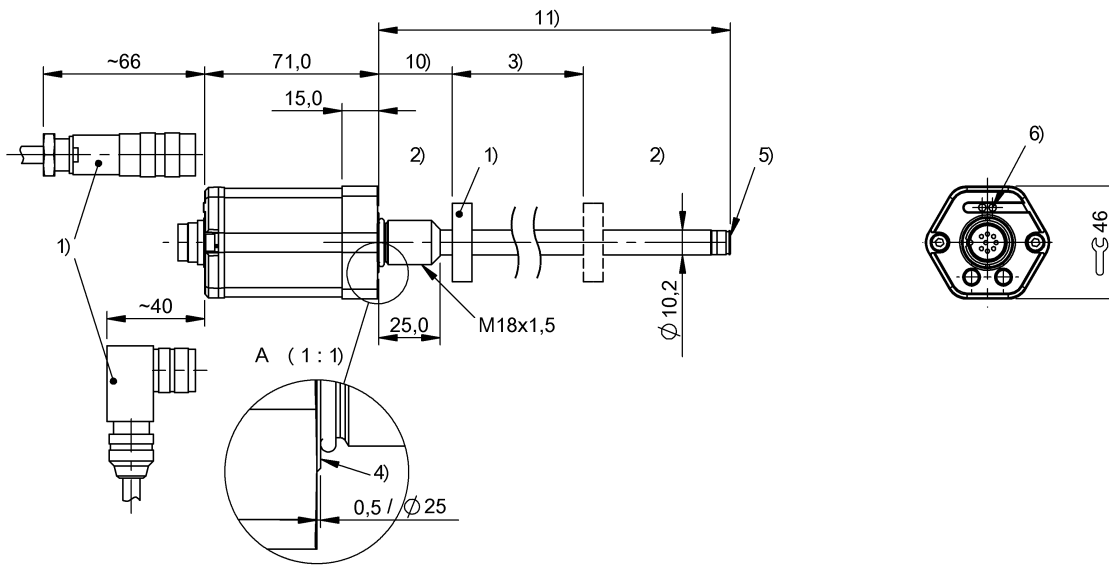
1) Не входит в комплект поставки 2) неиспользуемая область 3) Номинальная длина = измеряемая длина 4) Контактная поверхность 5) Внутренняя резьба M4x4/6 глубиная 6) Функциональный СИД 10) Нулевая точка 11) Монтажная длина
