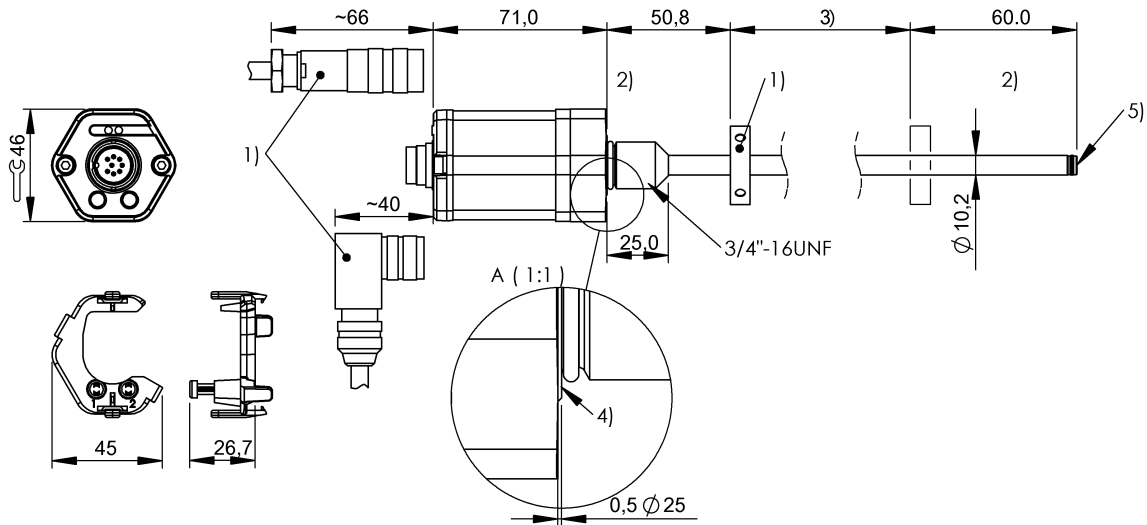
1) Не входит в комплект поставки 2) неиспользуемая область 3) Номинальная длина = измеряемая длина 4) Контактная поверхность 5) Внутренняя резьба M4x4/6 глубокая
