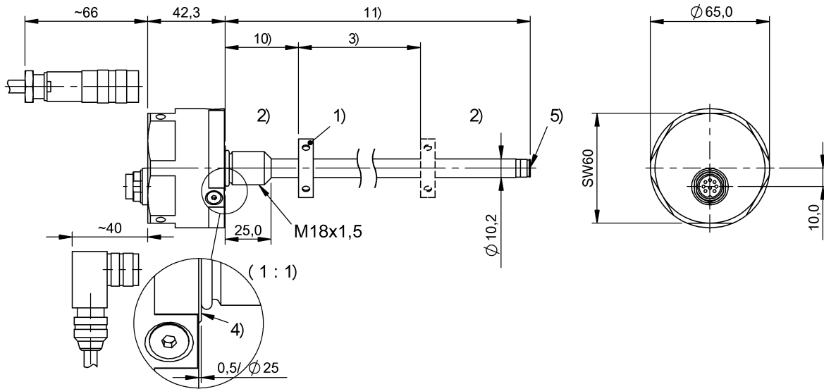
1) Не входит в комплект поставки 2) неиспользуемая область 3) Номинальная длина = измеряемая длина 4) Контактная поверхность 5) Внутренняя резьба M4x4/6 глубокая 10) Нулевая точка 11) Монтажная длина
