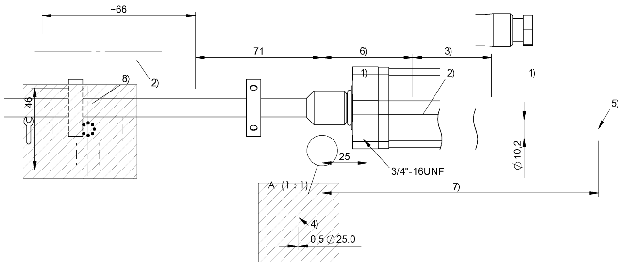
1) Не входит в комплект поставки 2) неиспользуемая область 3) Номинальная длина = измеряемая длина 4) Контактная поверхность 5) Внутренняя резьба M4x4/6 глубокая 6) Нулевая точка 7) Монтажная длина 8) Функциональный СИД
