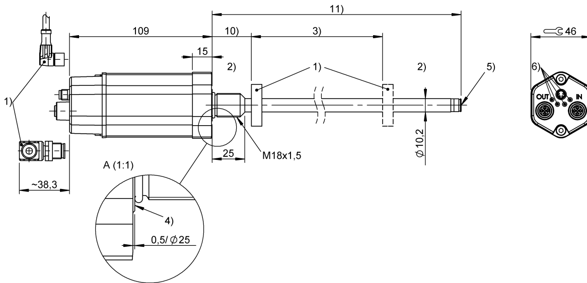
1) Не входит в комплект поставки 2) неиспользуемая область 3) Номинальная длина = измеряемая длина 4) Контактная поверхность 5) Внутренняя резьба M4x4/6 глубиной 5) Функциональный СИД 10) Нулевая точка 11) Монтажная длина
