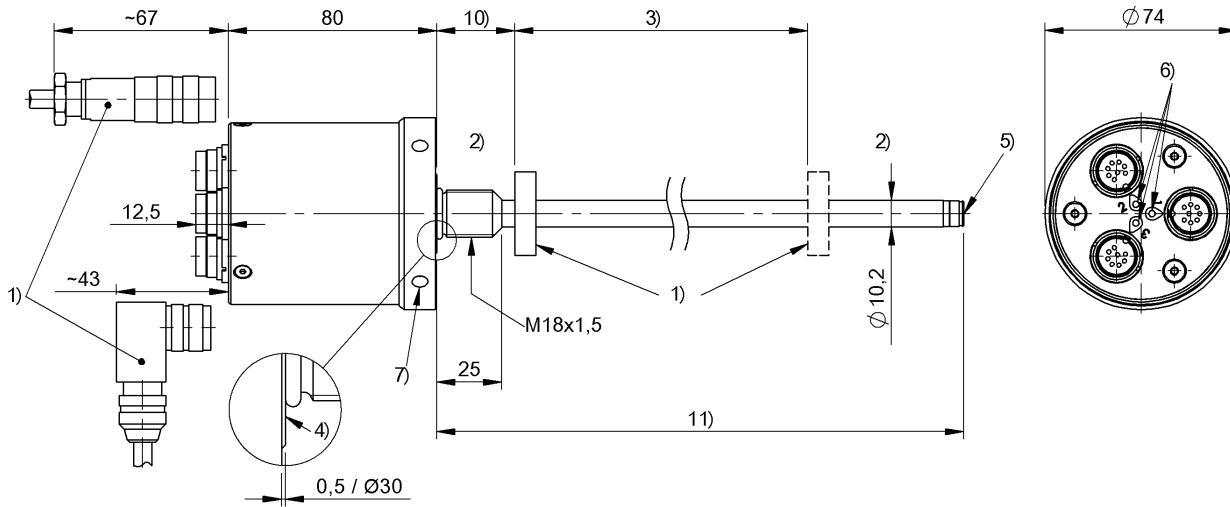
1) Не входит в комплект поставки 2) неиспользуемая область 3) Номинальная длина = измеряемая длина 4) Контактная поверхность 5) Внутренняя резьба M4x4/6 глубиной 6) Функциональный СИД 7) Ø6,1 под крючковый ключ Ø74 10) Нулевая точка 11) Монтажная длина
