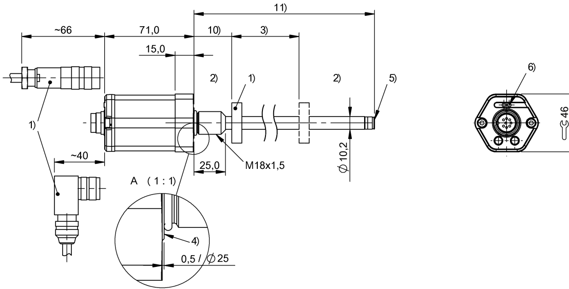
1) Не входит в комплект поставки 2) неиспользуемая область 3) Номинальная длина = измеряемая длина 4) Контактная поверхность 5) Внутренняя резьба M4x4/6 глубиная 6) Функциональный СИД 10) Нулевая точка 11) Монтажная длина
