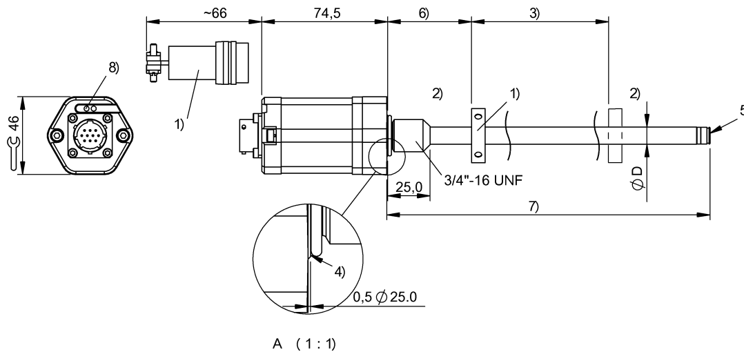
1) Не входит в комплект поставки 2) неиспользуемая область 3) Номинальная длина = измеряемая длина 4) Контактная поверхность 5) Внутренняя резьба M4x4/6 глубокая 6) Нулевая точка 7) Монтажная длина 8) Функциональный СИД
