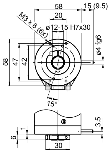
GXP5S - connector D-SUB
