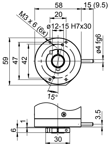
GXP5S - connector M23
