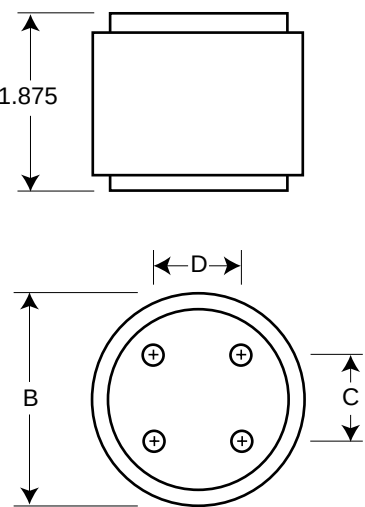
Fig. 2: 4000 Amp Range
