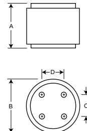
Fig. 3: 1500-2500 Amp Range
