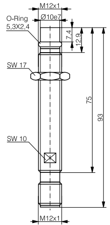
DW-AS-52#-P12-621
