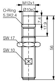
DW-AS-52#-P12-630
