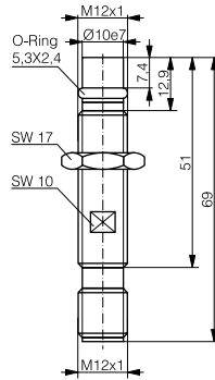
DW-AS-52#-P12
