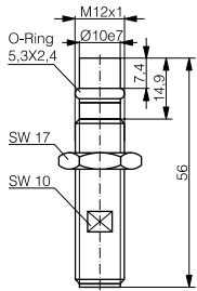
DW-AS-52#-P12-624
