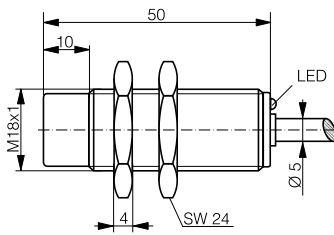
DW-AD-617/618-M18
