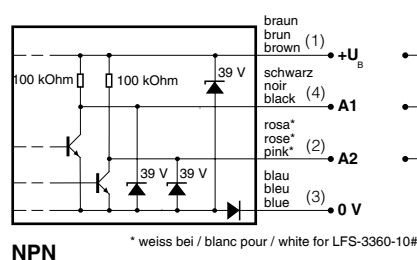
NPN
