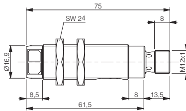
LLS-1180W-00#
