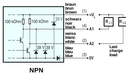
NPN
