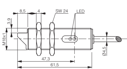
LLK-1180W-00#
