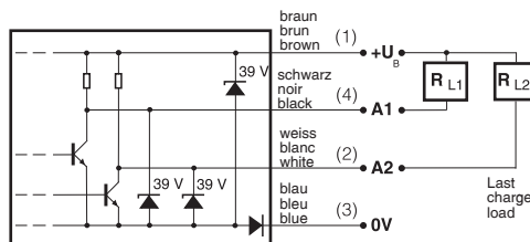
NPN
