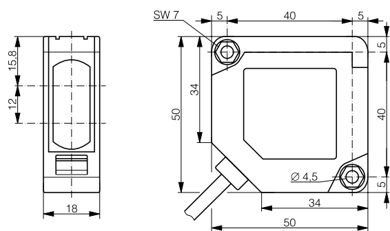
LTK-5050-10#
