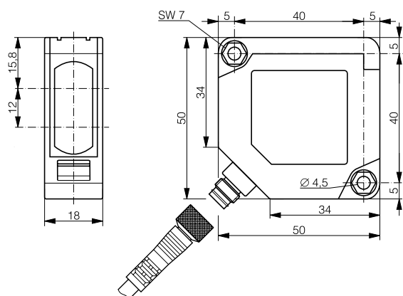
LTS-5050-10#
